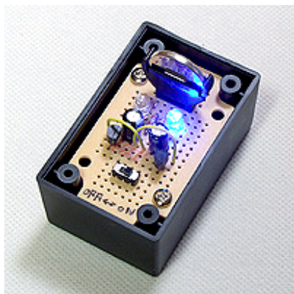
無安定マルチバイブレータ
